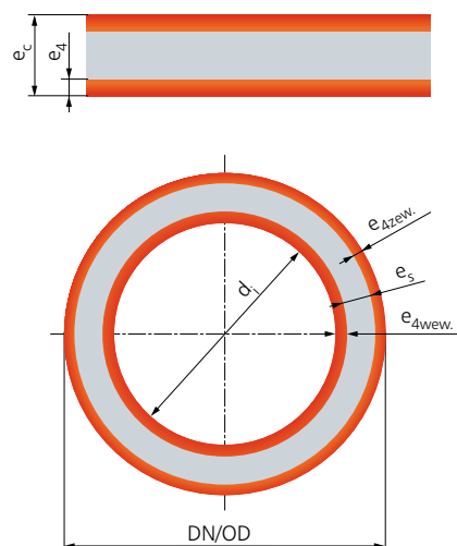
Przekrój rury strukturalnej z PVC-U typu A1
